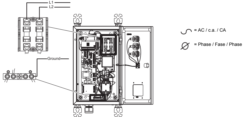
Figure / Figura / Figure 3 : Wiring Diagram / Diagrama de alambrado / Schéma de câblage
